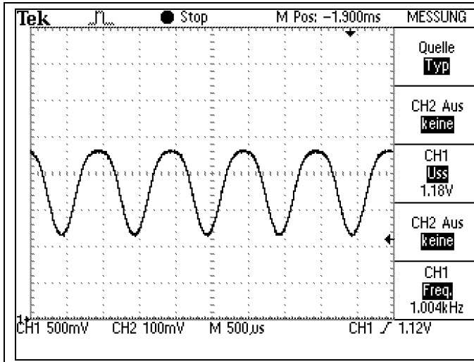
Bild 1 Das Oszillogramm zeigt ein konstantes Nutzsignal mit einem demodulierten 1 kHz-Anteil.
