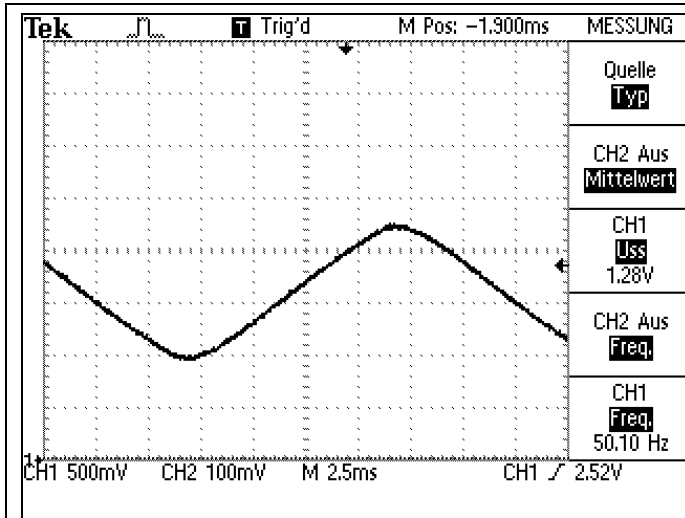
Bild 4 Nutzsinal ohne Beeinflussung
