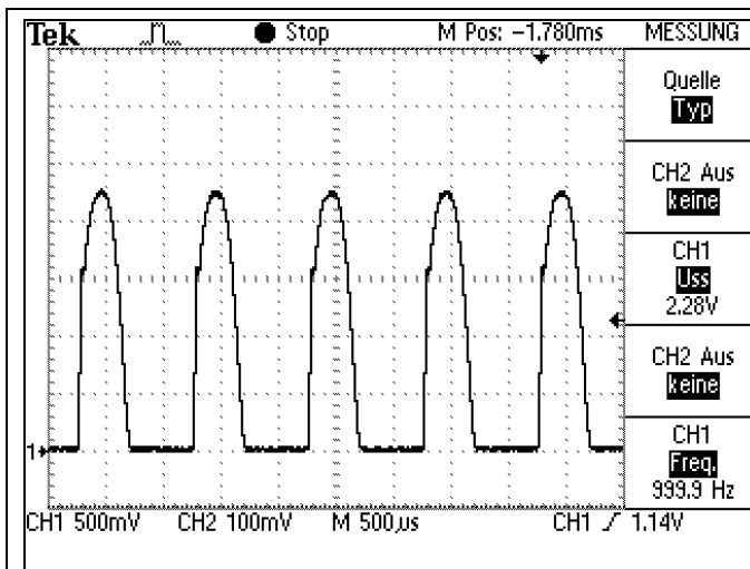
Bild 3 Das demodulierte 1 kHz-Störsignal wird von der unteren Schiene begrenzt.
