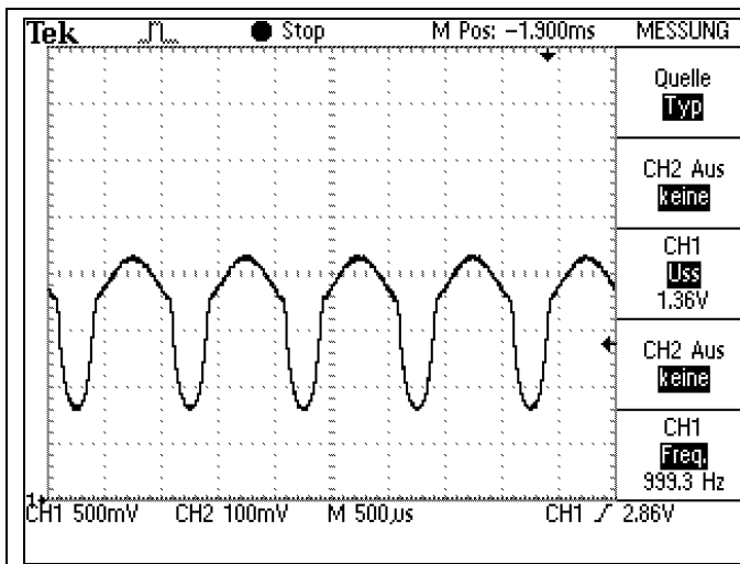
Bild 2 Das dem Nutzsignal überlagerte demodulierte 1 kHz-Störsignal zeigt hohen Oberschwingungsgehalt.
