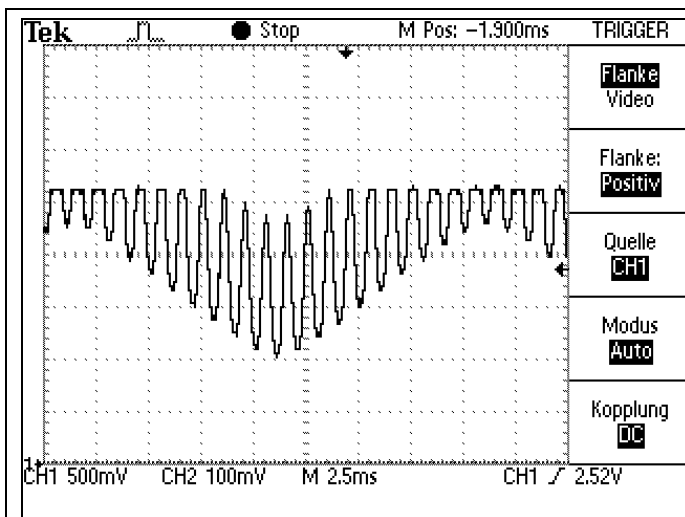
Bild 6 Nutzsinal mit 1 kHz Störsignal durch obere Schiene begrenzt
